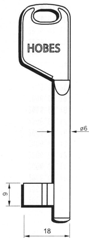
HOBES 36 ø6
