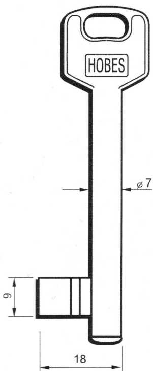
HOBES 36 ø7
